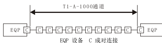
图1 T1-A-1000 信道组成
